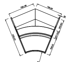
VBC 45 AA
