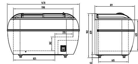
EHCDT (cabecera/end case)
