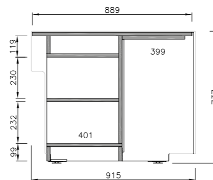
Sección comercial modelo MHD MHD model commercial section
