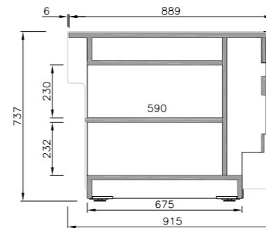
Sección comercial modelo M M mode commercial section
