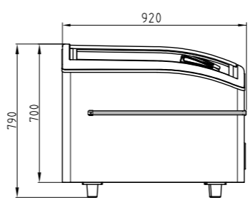
EHC MIXTO
