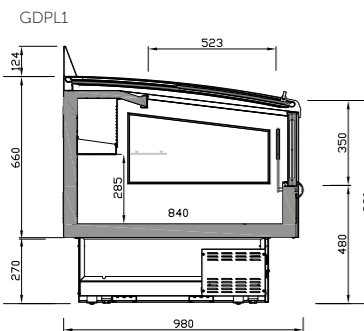
GDCPL1
