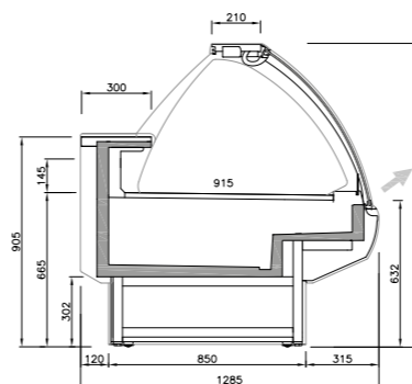
Sección comercial Commercial section Ángulos para módulos con reserva Angles for modules with reservation
