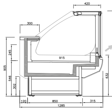
Sección comercial Commercial section Ángulos para módulos sin reserva Angles for modules without reservation
