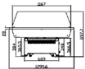
Perfil Profile
